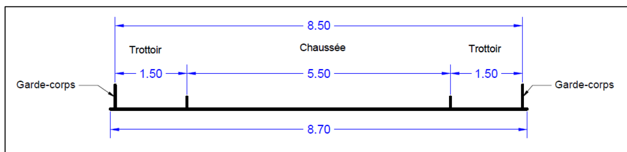
Figure 2 : Coupe fonctionnelle courante sur l'ouvrage existant
