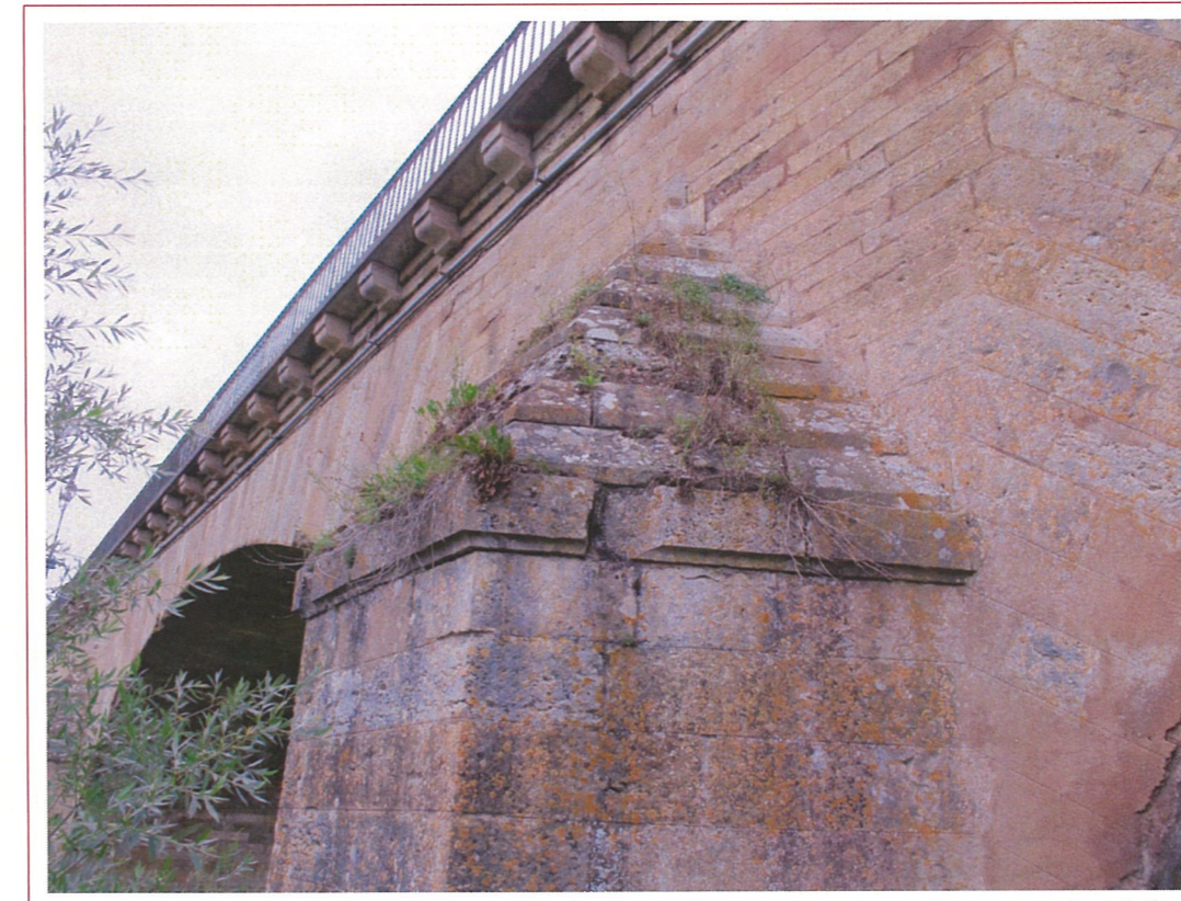
Arrière bec Pile 3 Epaufure -Photo 21-
