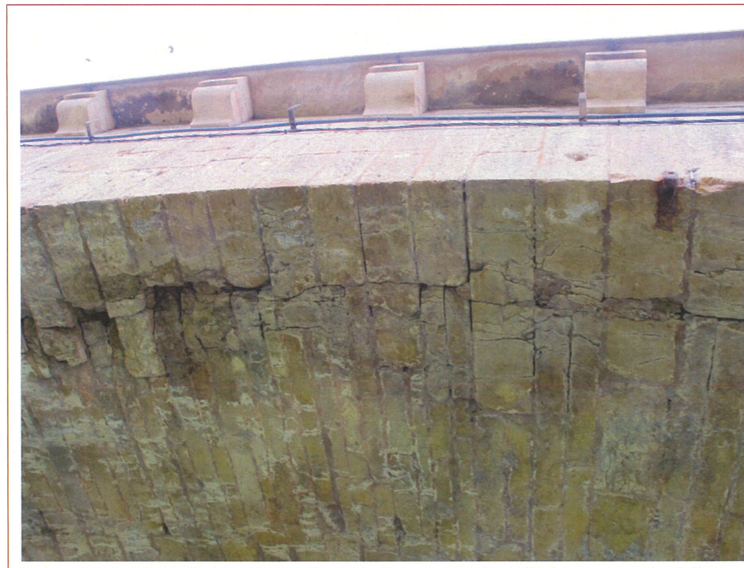
Vue de la voûte en aval de la passe 8 Fracture annulaire et érosion -Photo 52-
