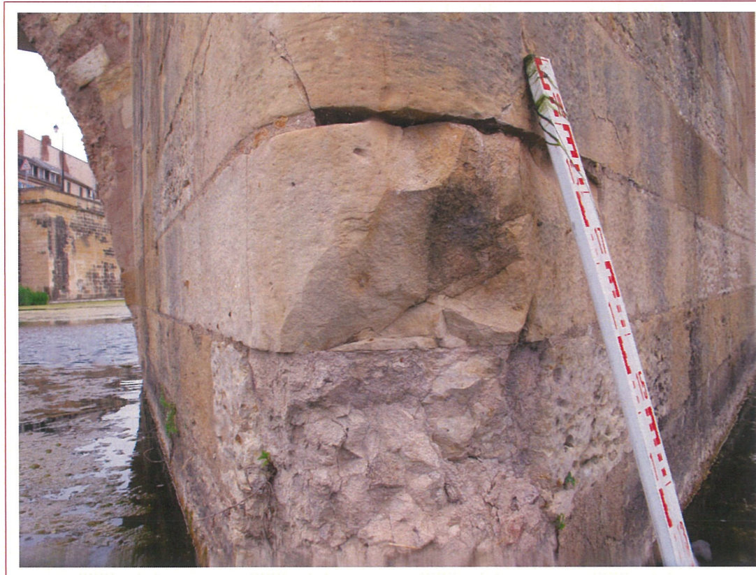
Avant bec Pile 1 Epaufrement et érosion -Photo 8-
